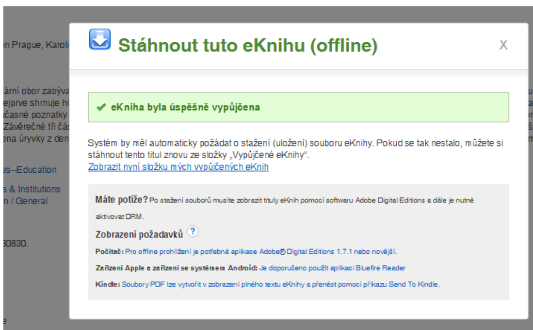
Obr. 8 Offline výpůjčka
